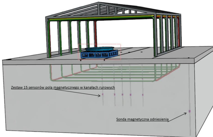
Rysunek 1. Zobrazowane stanowisko pomiarowe
